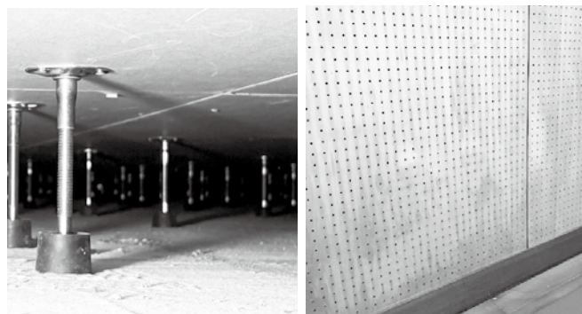
写真2：床の防音
